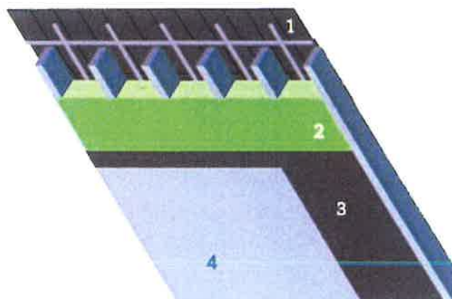
1. Onderdak | 2. Isolatie | 3. Dampscherf | 4. binnenafwerking
